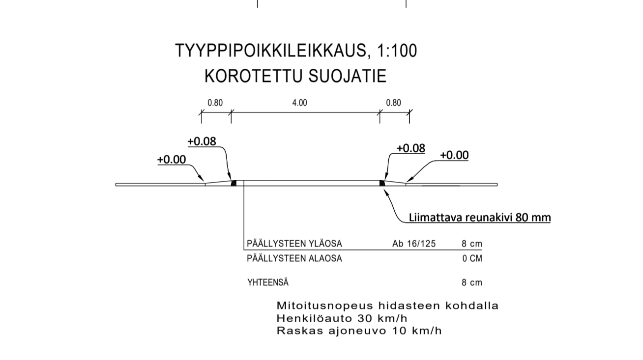
TYYPPIKOIKKEIKKAUS, 1:100 KOROTETTU SUOJATIE
