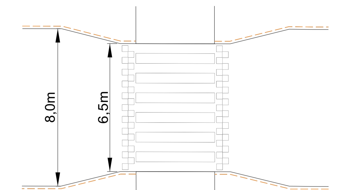
TASOKUVA, 1:100 SUOJATIE KAVENNUS JA KOROTETTU SUOJATIE, KOULUKATU
