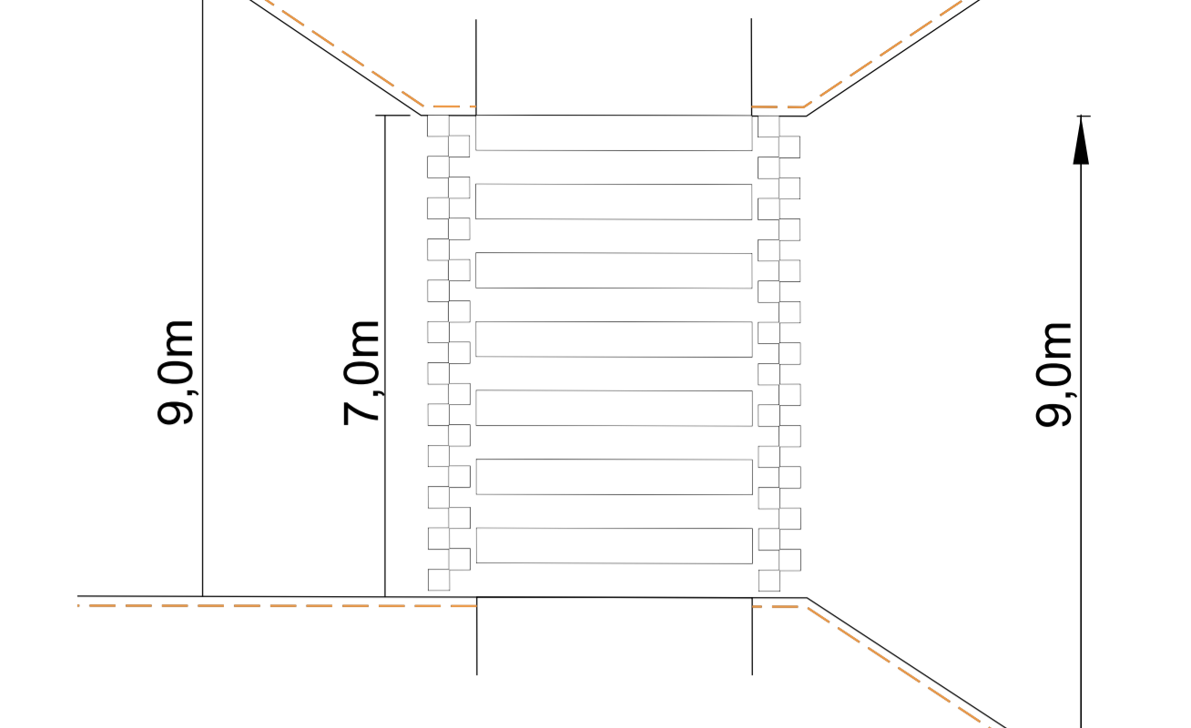
TASOKUVA, 1:100 SUOJATIE KAVENNUS JA KOROTETTU SUOJATIE, KOULUKATU
